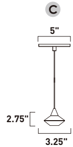
E25028-BKPC, -WTPC Pendant
