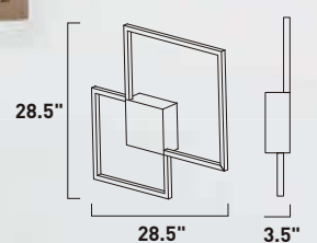
E21510-CHP Wall Mount D
