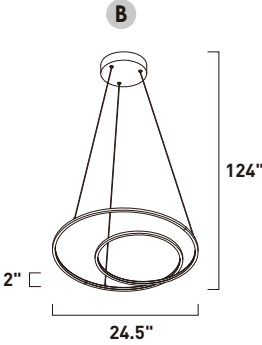
E21325-BK, MS Pendant
