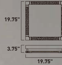
E21230-MW Flush Mount
