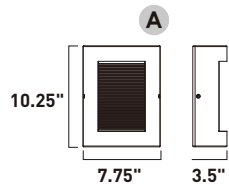
E14380-GSN, SSN Interior/Exterior Wall Sconce
