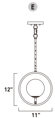
E12519-92PN Mini Pendant
