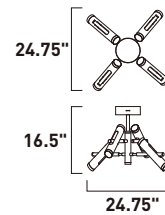
E25044-BKSN Flush Mount
