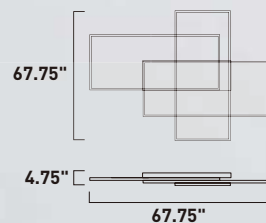
E21519-BK, CHP Flush Mount E
