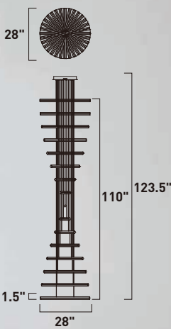
E21379-BK Pendant A
