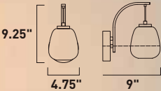
E25060-92BKGLD Wall Mount
