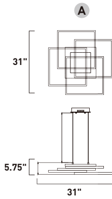
E21516-BK, CHP Pendant
