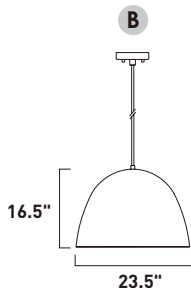
E24916-BKSBR, -DGCOF, -SNBK Pendant
