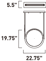
E24081-NAB Pendant B
