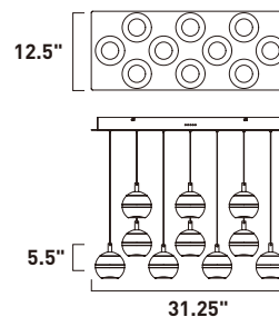
E24599-93NAB, -93PC Pendant
