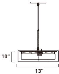
E51011-BKGLD, -WT, -WTBK, -WTGLD Pendant
