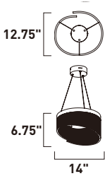
E24771-133BK Pendant B
