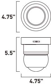
E23510-AL, -BK, -GLD Flush/Wall Mount
