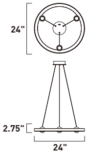
E23512-AL, -BK, -GLD Pendant
