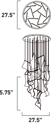
E24877-133PC, -133BGM Pendant
