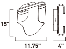
E24770-133BK Wall Mount C
