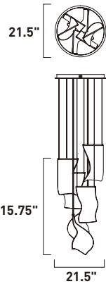
E24875-133PC, -133BGM Pendant A
