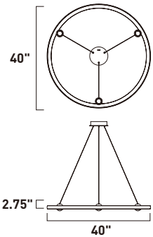
E23514-AL, -BK, -GLD Pendant A
