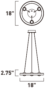
E23511-AL, -BK, -GLD Pendant
