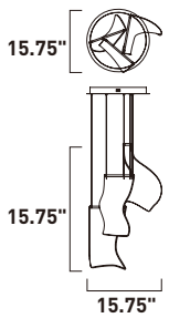
E24874-133PC, -133BGM Pendant B
